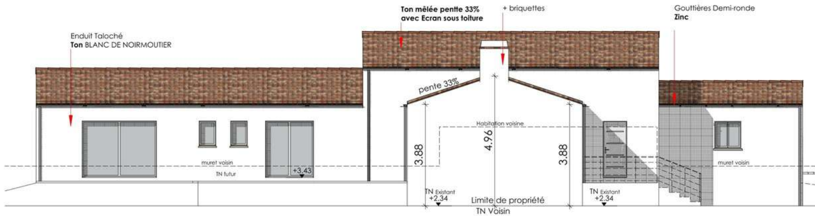
FACADE SUD-EST
